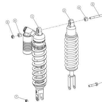
LP24 - AMORTECEDOR – TRASEIRO / REAR SHOCK ABSORBER
